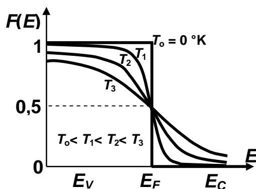
Fig. 4.5 – Funzione di Fermi
