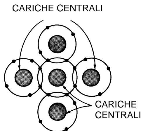
Fig. 4.2 – Legami covalenti in un cristallo di silicio
