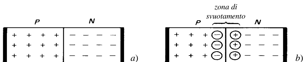
Fig. 4.10 – Giunzione p-n : a) prima della diffusione; b) dopo la diffusione
