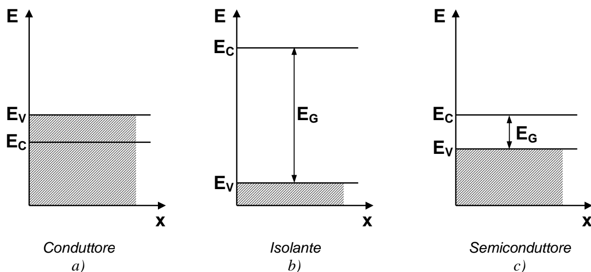
Fig. 4.4 – Distribuzione delle bande di valenza (di cui E_V è l'estremo superiore) e di conduzione (di cui E_C è l'estremo inferiore) in un a) conduttore, b) isolante, c) semiconduttore
