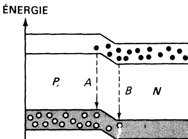
Fig. 4.12 – Ricombinazione in una giunzione polarizzata direttamente
