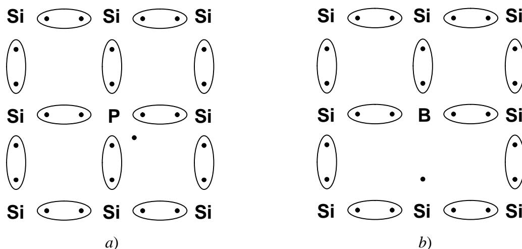
Fig. 4.7 – Cristallo di silicio drogato con: a) fosforo (tipo n), b) boro (tipo p)
