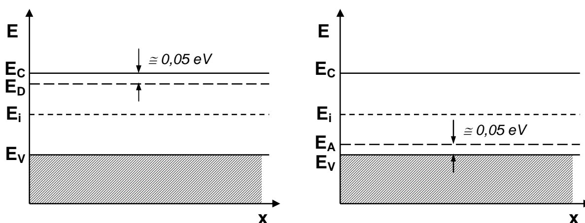
Fig. 4.8 – a) livello donatore in un semiconduttore di tipo n b) livello accettore in un semiconduttore di tipo p
