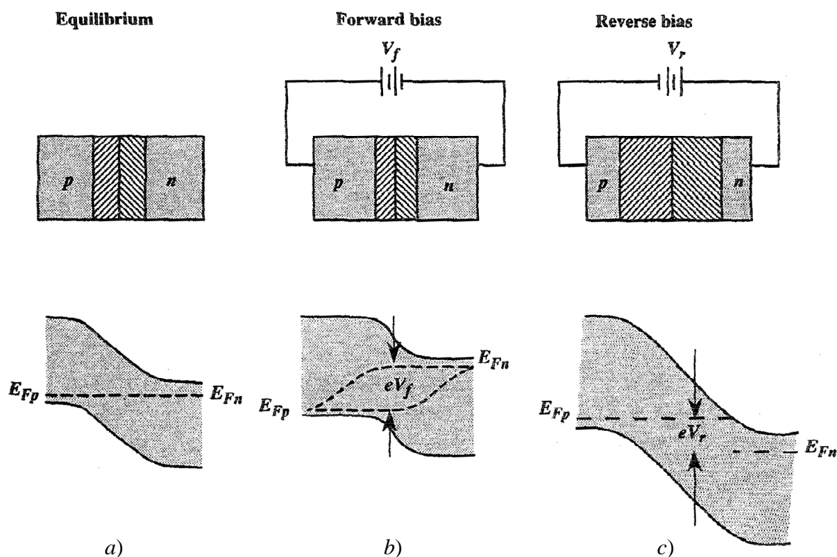
Fig. 4.11 – Bande di energia in una giunzione p-n a) all’equilibrio; b) polarizzata direttamente; c) polarizzata inversamente
