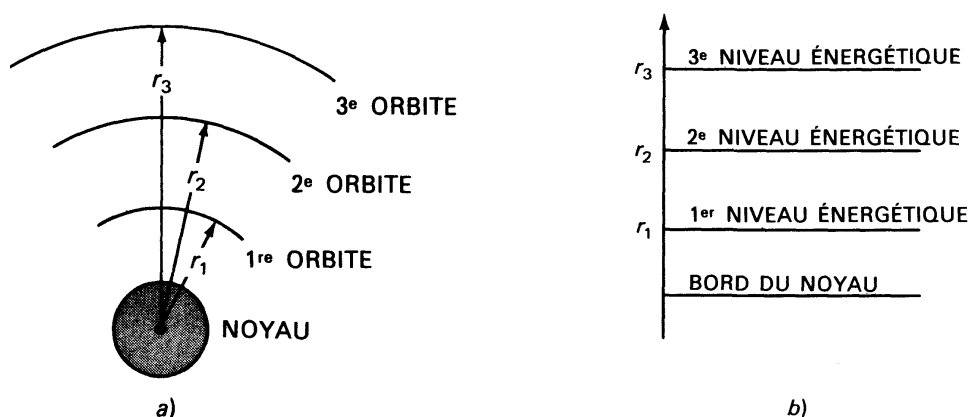
Fig. 4.1 – a) Schema di un atomo secondo Bohr. b) Livelli energetici
