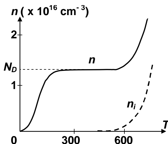
Fig. 4.9 – Andamento della concentrazione di elettroni in un semiconduttore di tipo n al variare della temperatura
